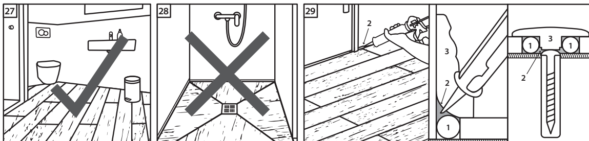
1: PE foam baker rod / PE Schaum Band, 2: Silicone / Silikon, 3: Molding / Leiste
