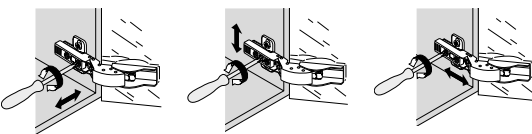
Justering i sidled. Justering i höjddled. Justering i djupled.
