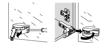
Demontering av gångjärn. Montering av gångjärn.
