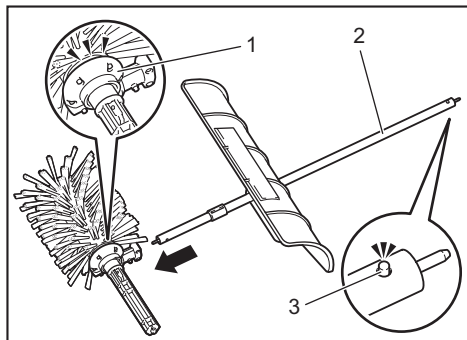
► 1. Reduktor 2. Toru 3. Tihvt
