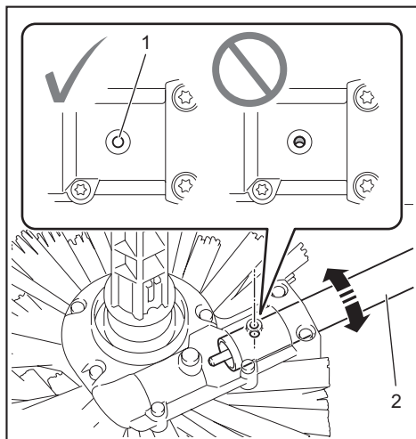
► 1. Hål 2. Rör
