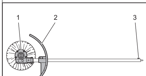
► 1. Pievada korpus 2. Aizsargs 3. Tapa
