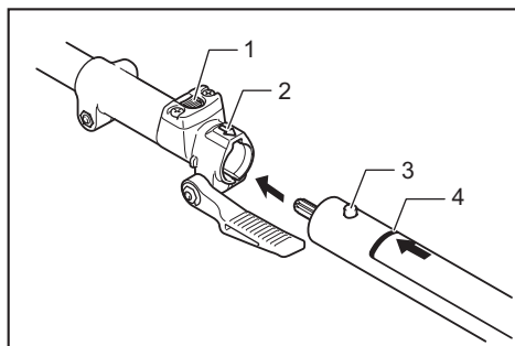
► 1. Vabastusnupp 2. Noolemärk 3. Tihvt 4. Asendijoon
