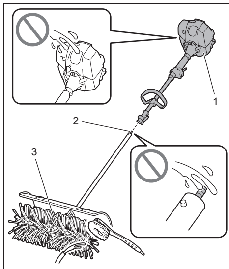
► 1. Drivverk 2. Rørende 3. Spindelkasse
