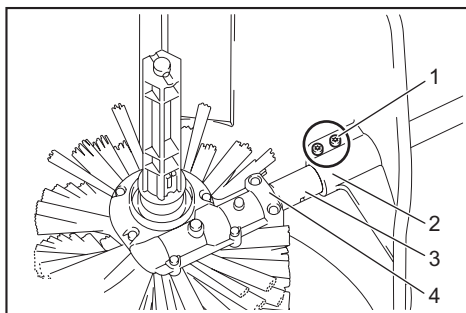
► 1. Ruuvi 2. Suojuks 3. Holkki 4. Hammasrattaisto
