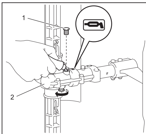
► 1. Polt 2. Reduktor
