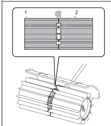
► 1. Подметальный барабан 2. Корпус редуктора
