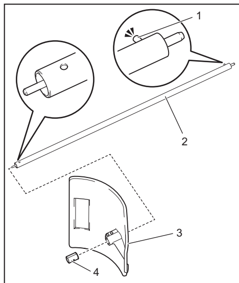
► 1. Stift 2. Rör 3. Skydd 4. Hylsa
