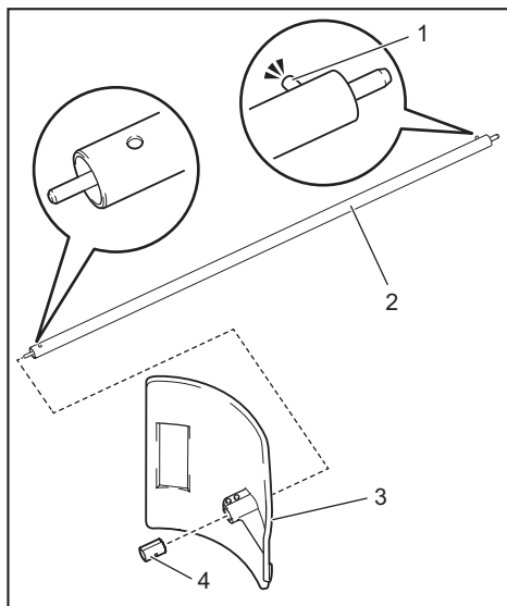
► 1. Tapa 2. Caurule 3. Aizsargs 4. Uzmava
