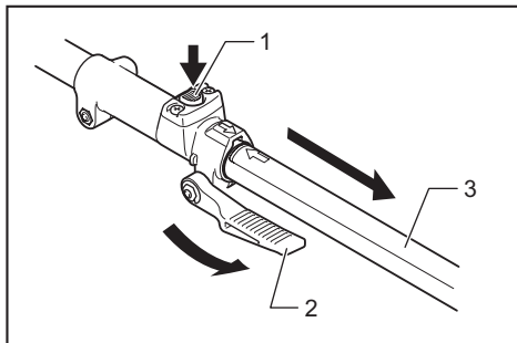
► 1. Atlaisvinimo mygtukas 2. Svirtis 3. Vamzdis
