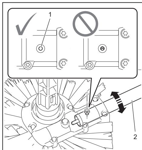
► 1. Отверстие 2. Трубка
