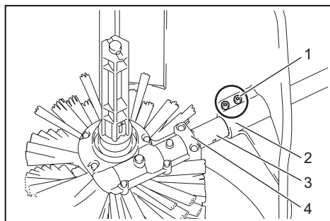
► 1. Kruvi 2. Kaitse 3. Hülss 4. Reduktor
