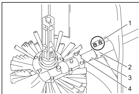
► 1. Skru 2. Vern 3. Hylse 4. Spindelkasse
