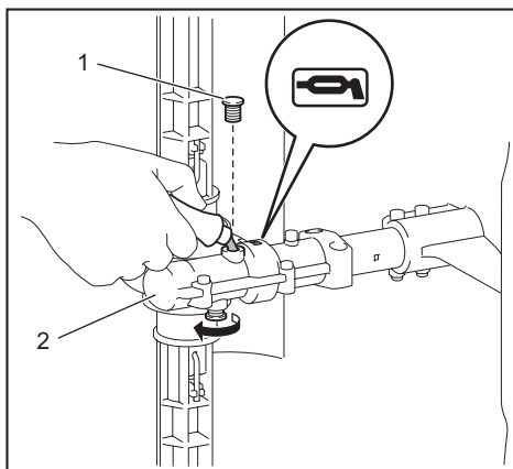
► 1. Bult 2. Växellåda
