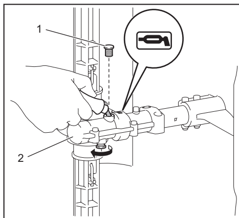
► 1. Pultti 2. Hammasrattaisto
