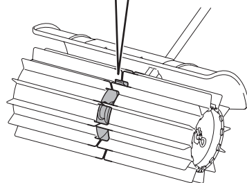
► 1. Pühkimistrummel 2. Reduktor
