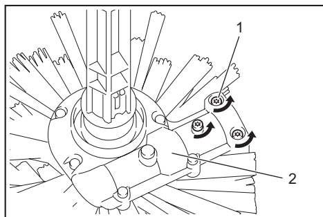
► 1. Ruuvi 2. Hammasrattaisto
