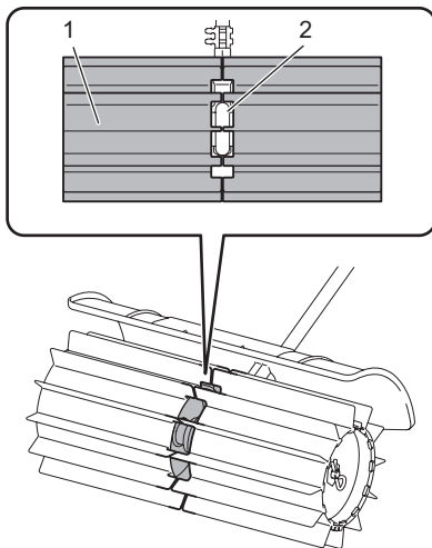
► 1. Sweep drum 2. Gear case
