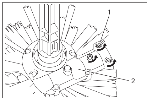
► 1. Skrūve 2. Pievada korpusss
