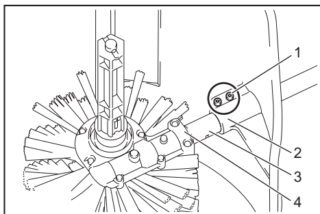
► 1. Varžtas 2. Apsauginis gaubtas 3. Įvorė 4. Pavarų dėžė
