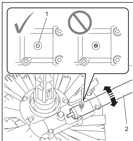
► 1. Anga 2. Vamzdis
