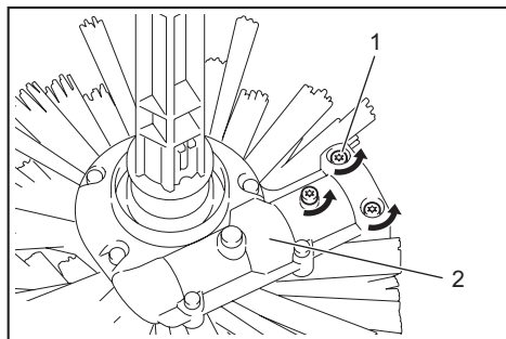
► 1. Skruer 2. Spindelkasse
