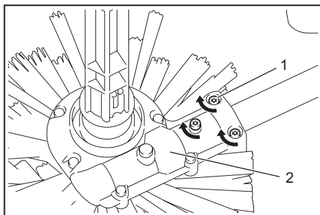
► 1. Skrūve 2. Pievada korpus
