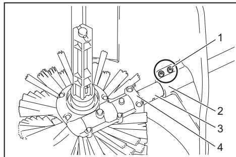
► 1. Винт 2. Защитный кожух 3. Ниппель 4. Корпус редуктора
