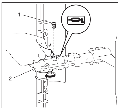
► 1. Skrūve 2. Pievada korpuss
