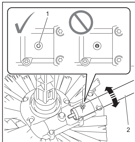
► 1. Hole 2. Pipe
