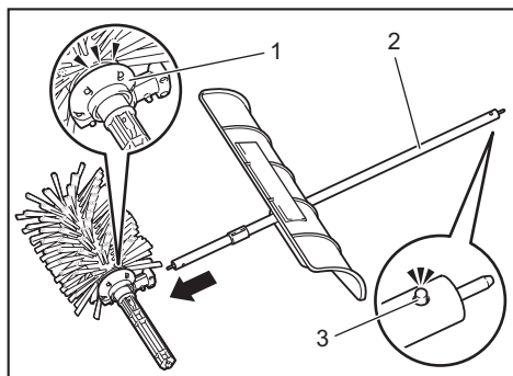
► 1. Pavarų dėžė 2. Vamzdis 3. Smaigas
