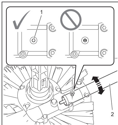
► 1. Caurums 2. Caurule
