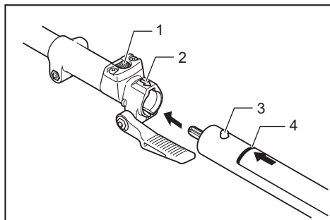
► 1. Atlaišanas poga 2. Bultiņas atzīme 3. Tapa 4. Novietojuma līnija
