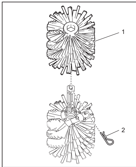
► 1. Hari 2. Klamber
