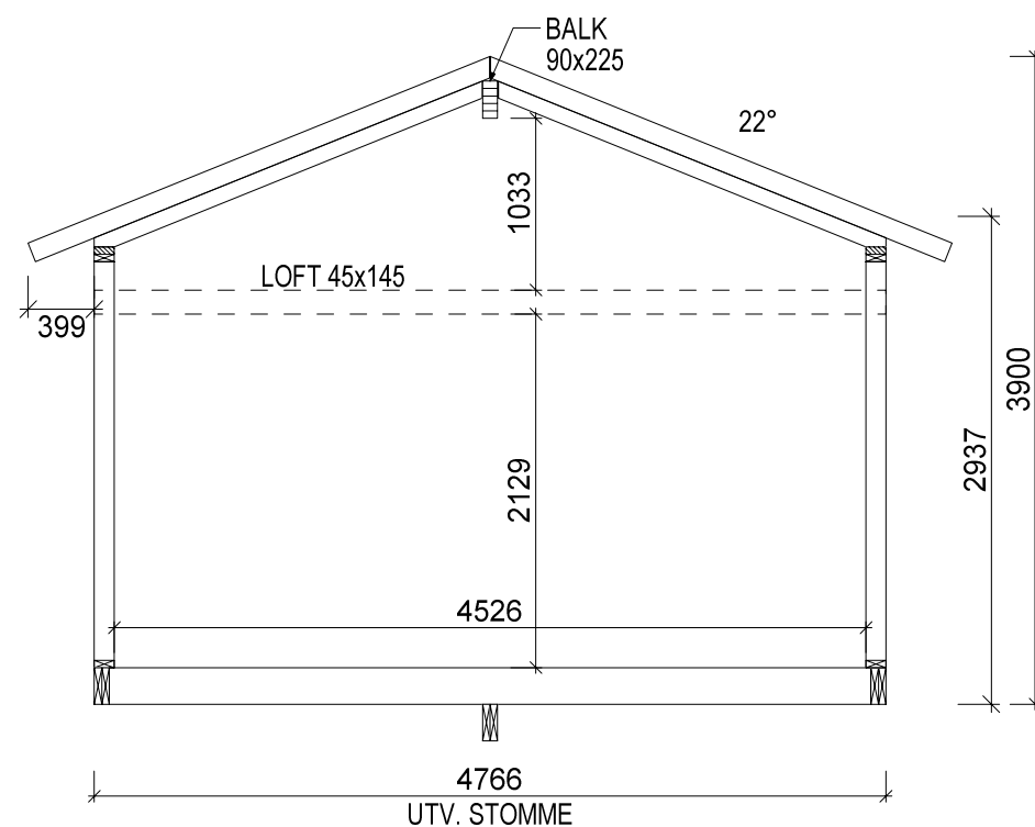
SEKTION B-B
