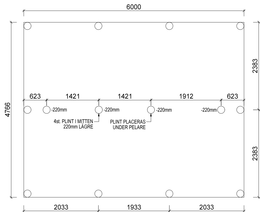
PLINTGRUND
