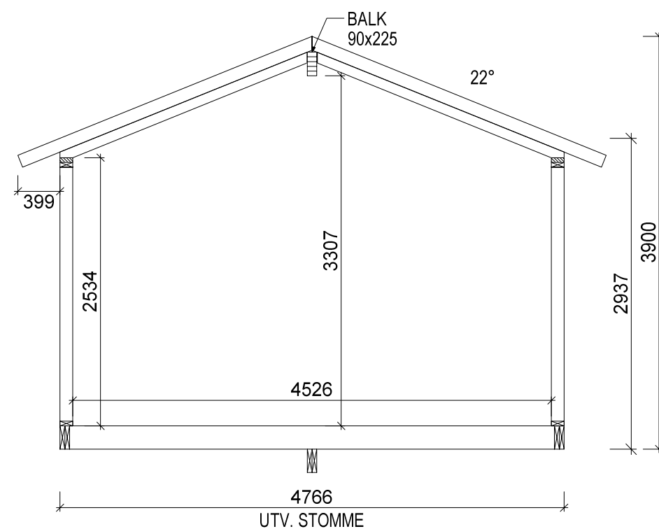
SEKTION A-A
