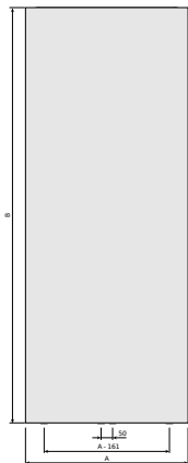
Paros V, typ 21, frontvy
