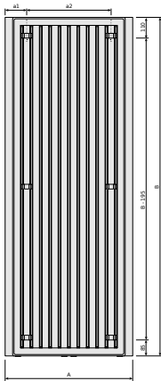
Paros V, bakvy
