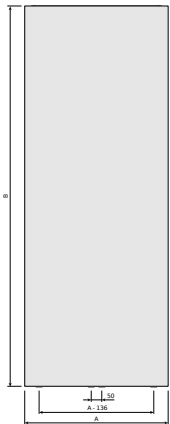
Paros V, typ 11, frontvy
