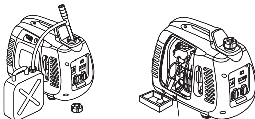
Tyhjennysruuvi
