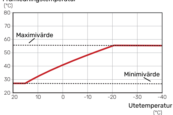
Framledningstemperatur
