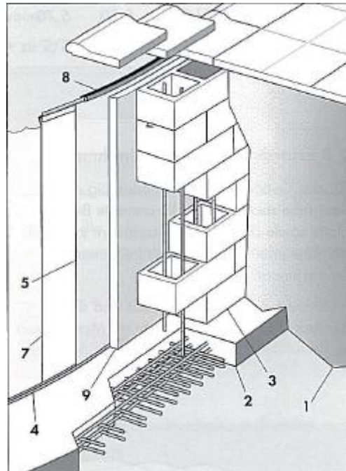
(1) Jordmån, (2) Armerad bottenplatta, (3) Armerad stödmur, (4) Bottenskena, (5) Stålmantel, (7) Liner, (8) Räcke, (9) Isolering, (11) Fastsättningsvinkel
