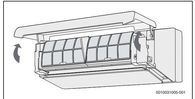
Bild 16 Demontera frontluckan
