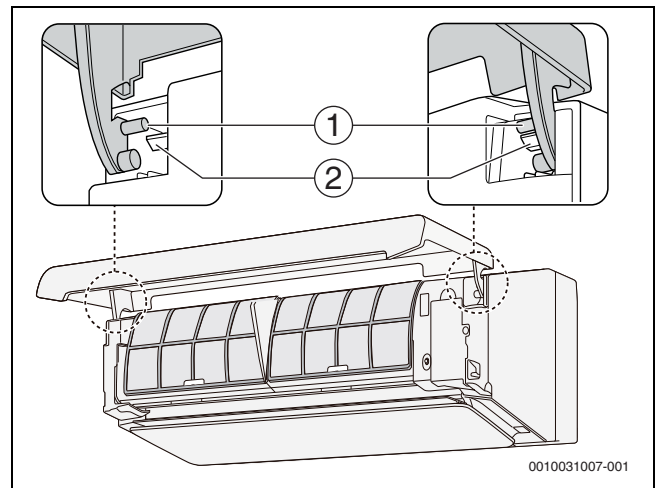
Bild 18 Demontera lucka
