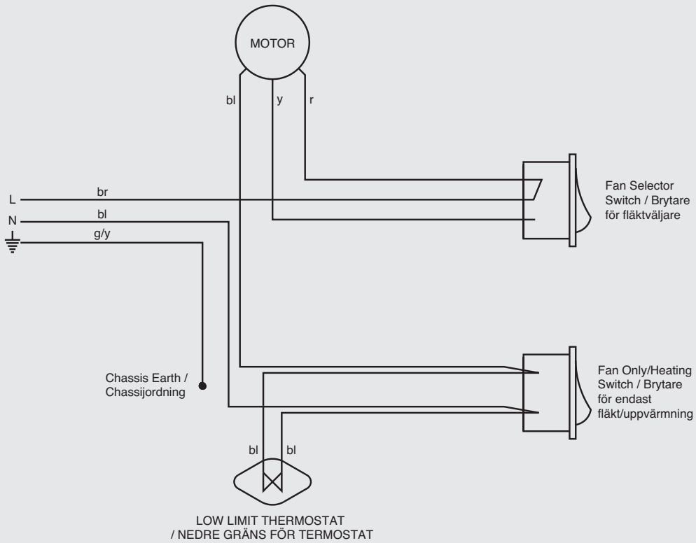
Fig. 7a KICKSPACE® 500, 600, 800, 80S & 80D wiring diagram / Kopplingschema för KICKSPACE® 500, 600, 800, 80S och 80D
