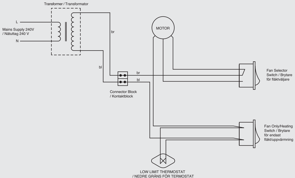
Fig. 7b KICKSPACE® 600-12V wiring diagram / Kopplingschema för KICKSPACE® 600-12V
