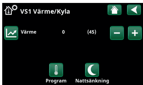
Meny "Avancerat/Definiera/Värmesystem/Värmesystem 1". Värmesystemet saknar rumsgivare. Inom parentes visas börvärdet (framledningstemperatur 45\text{ }^{\circ}\text{C} ). Till vänster om börvärdet visas utomhustemperaturen ( 0\text{ }^{\circ}\text{C} ) vid aktuell framledningstemperatur.
