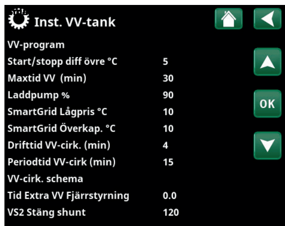
Del av meny "Avancerat/Inställningar/Varmvatten"
