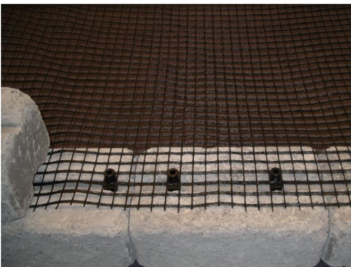
Bild 3. Montering av Bender Geonät på första skiftet. Sätt fast nätet över låspluggarna. Låt pluggarna sticka upp ur tredje raden på nätet så att så mycket nät som möjligt ligger mellan stenlagren utan att sticka ut. Då sitter nätet bäst.
