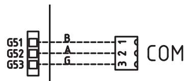
Detaljbild från elschemat
