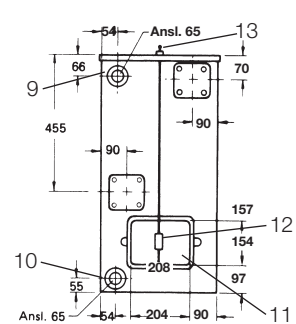
Baksektion
