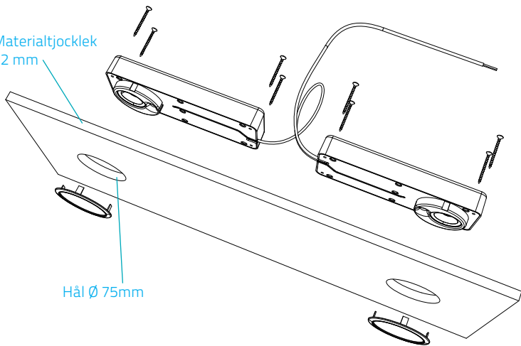
Montage inifrån
