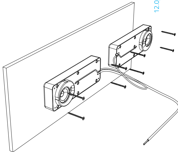
Montage utifrån
