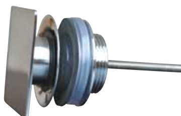
Pop-up ventil Fyrkantig plan propp. Förkromad mässingsöver- och underdel. Utv. R32. Art nr 857 35 77
