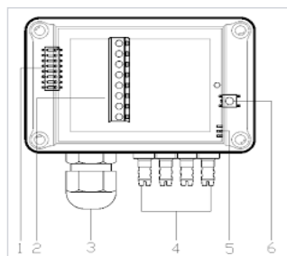
art.nr: 340097 Trycktransmitter QBM 68.2525
