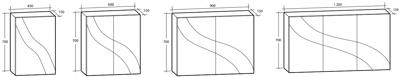
Spegelskåp Ella 45
