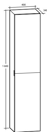
Högskåp 2Day 400
