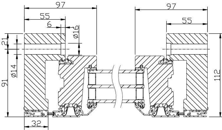
Horizontalsnitt bågpost
