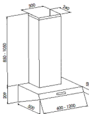
Måttskiss
