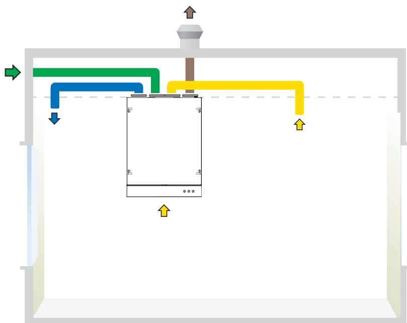
CASA R2 R, högerutförande Spiskåpa Jazz
