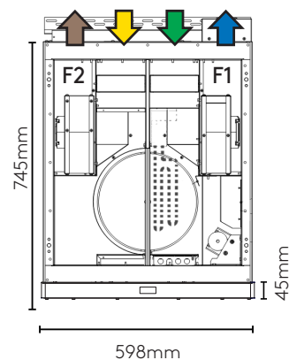
CASA R2 R, högerutförande Spiskåpa Dance
