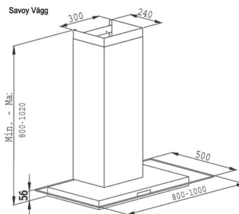
Måttskiss
