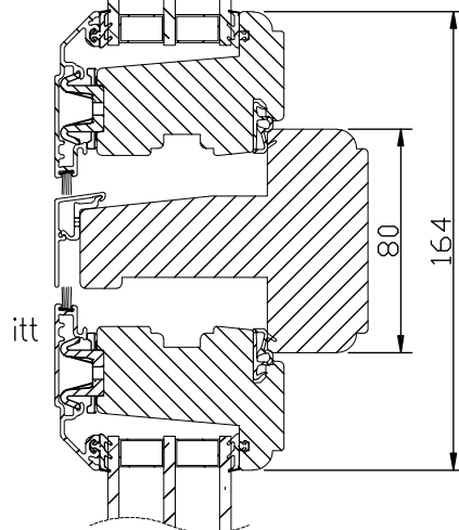
Vertikalsnitt karm tvärpost
