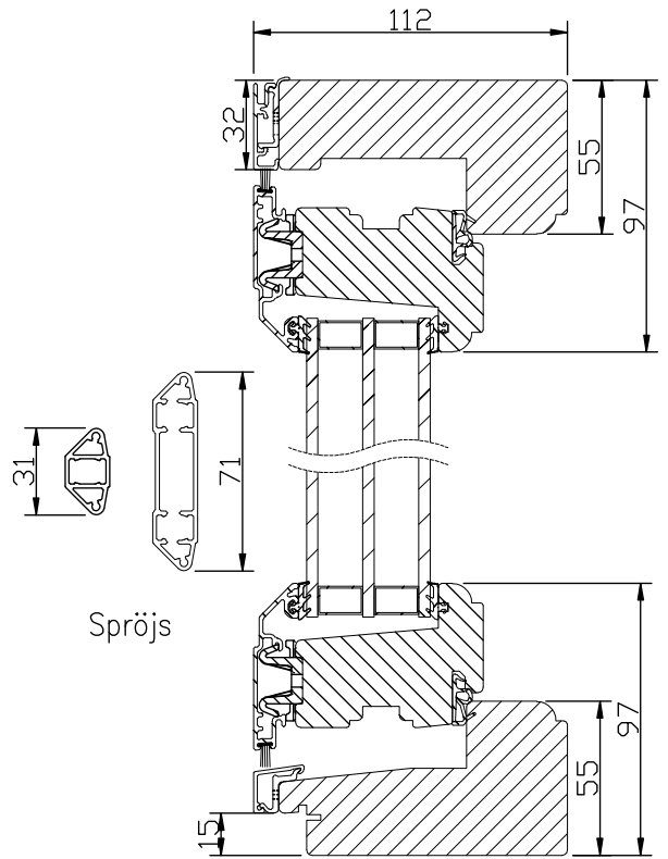
Vertikalsnitt
