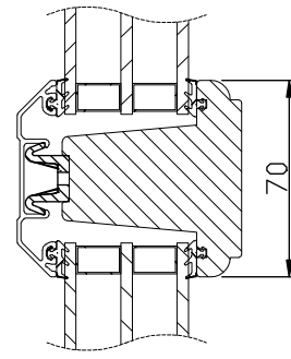
Vertikalsnitt bågpost
