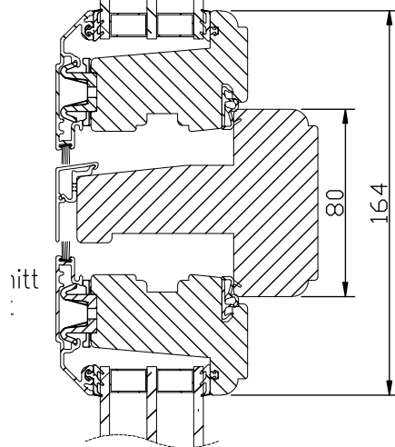
Vertikalsnitt karm tvärrast
