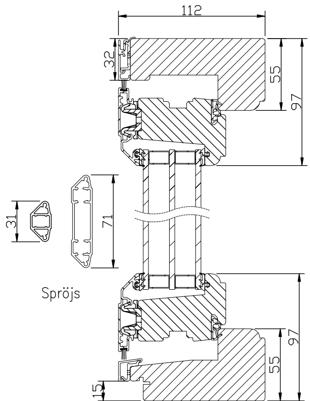
Vertikalsnitt
