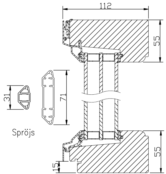
Vertikalsnitt
