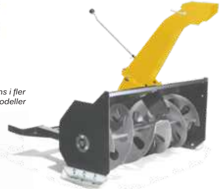
Snöslunga 2-steps (Park 740 IOX). Det hydrauliskt kontrollerade inmatningshuset samlar in snön och kastar den upp till 12 m från utkastet. Finns i fler utföranden anpassade för andra modeller av Stiga Park.
