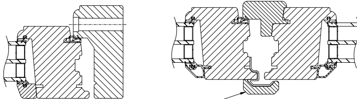
Horizontalsnitt pardörr
