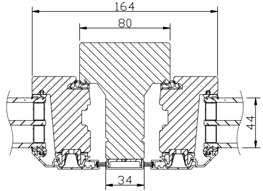
Horizontalsnitt
