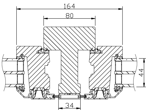
Horizontalsnitt karm mittpost
