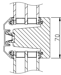
Vertikalsnitt bågpost
