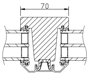
Horizontal bågpost
