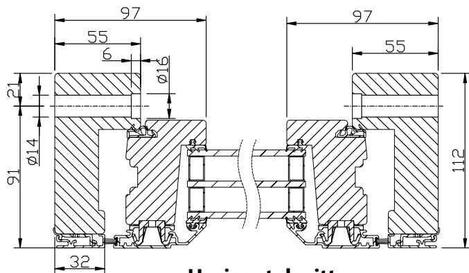
Horizontalsnitt
